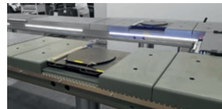
Drehteller und Ausgleichsstücke fixiert mit Zahnleiste
