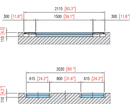
Optional auch mit mobilem Rahmen für die vollige Unabhängig erhältlich Option mobil kit frame
